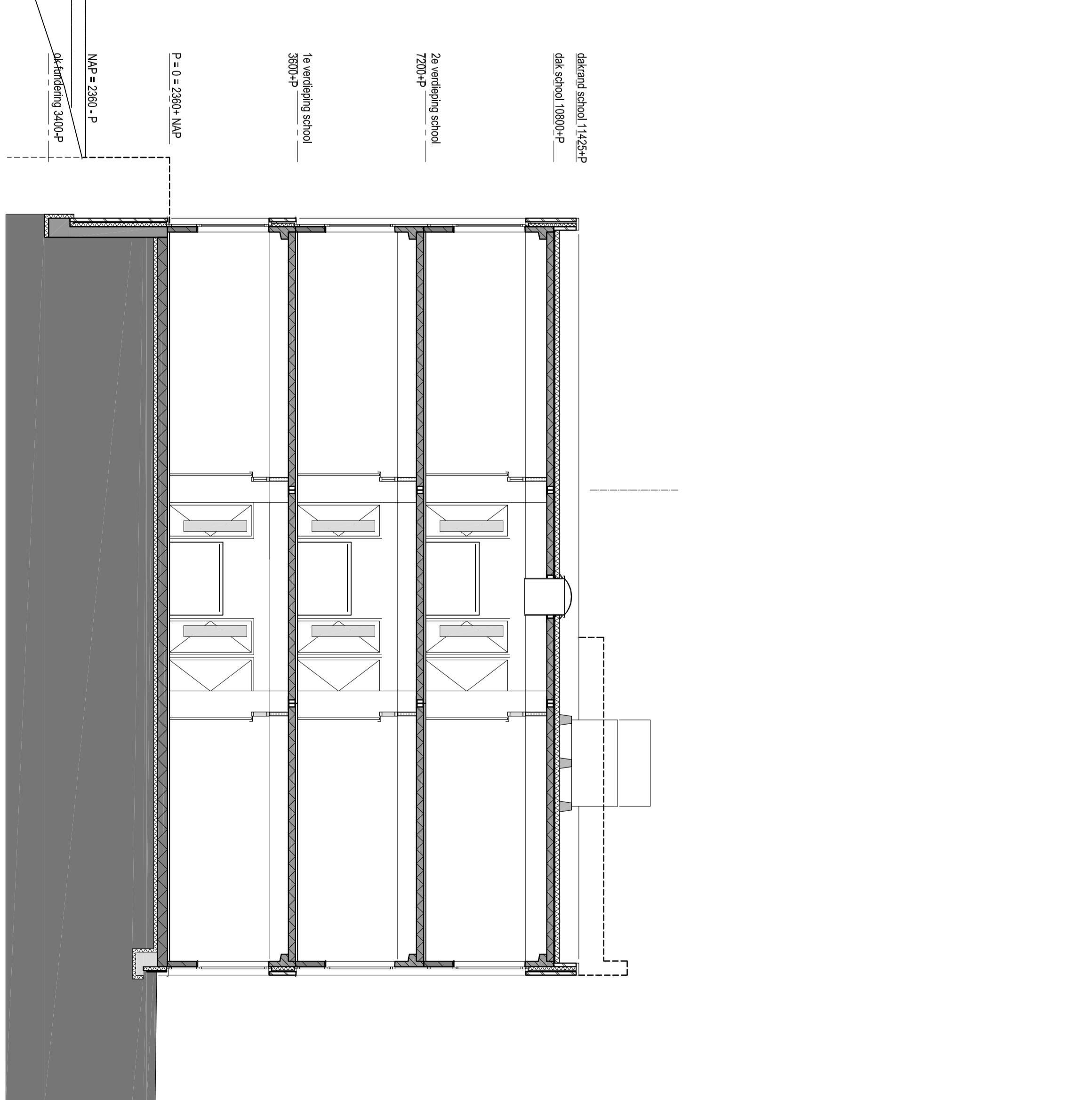
doorsnede 5-5
