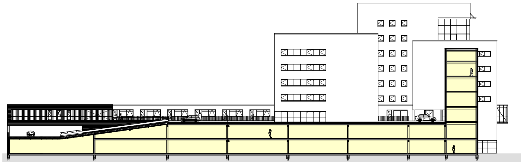
LANGSDOORSNEDE
