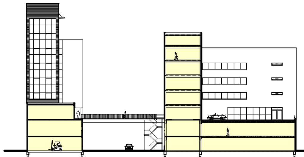
DWARSDOORSNEDE
