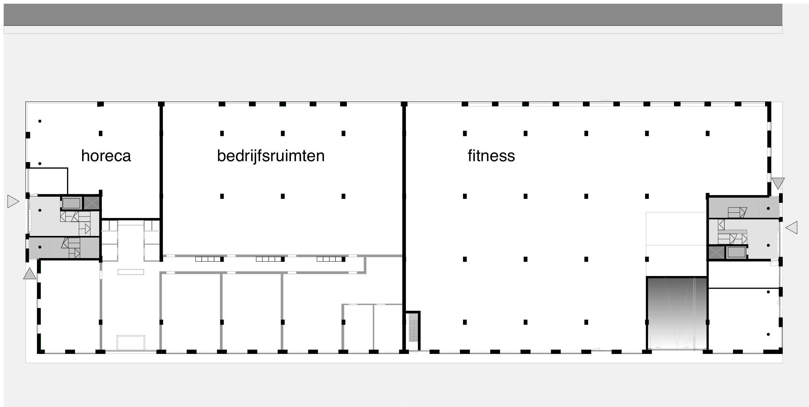
begane grond
