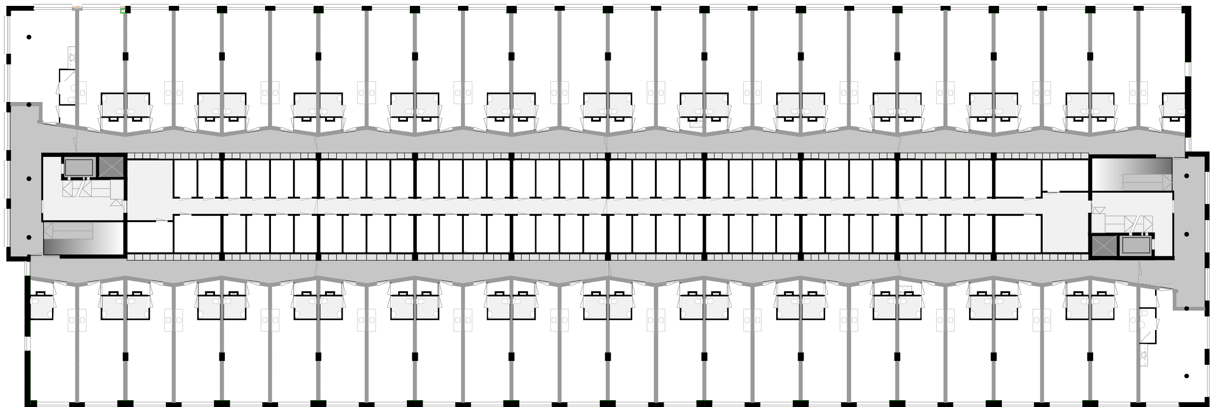
1e verdieping
