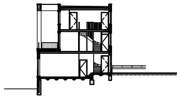
Doorsnede type 3
