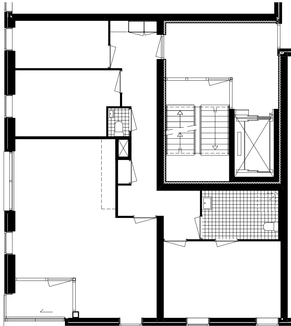
Woningtype G1s
