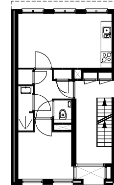
Type F 1e Verdieping
