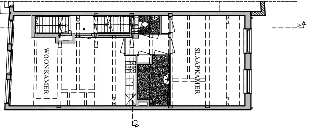
woning 2 1e VERDIEPING NR. 32
