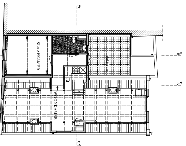
woning 1 BELETTAGE NR. 34 BEGANE GROND NR. 32
