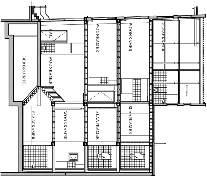
DOORSNEDEN B-B
