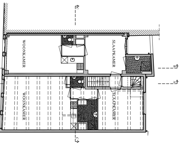
woning 1 SOUTERRAÏN NR. 34
