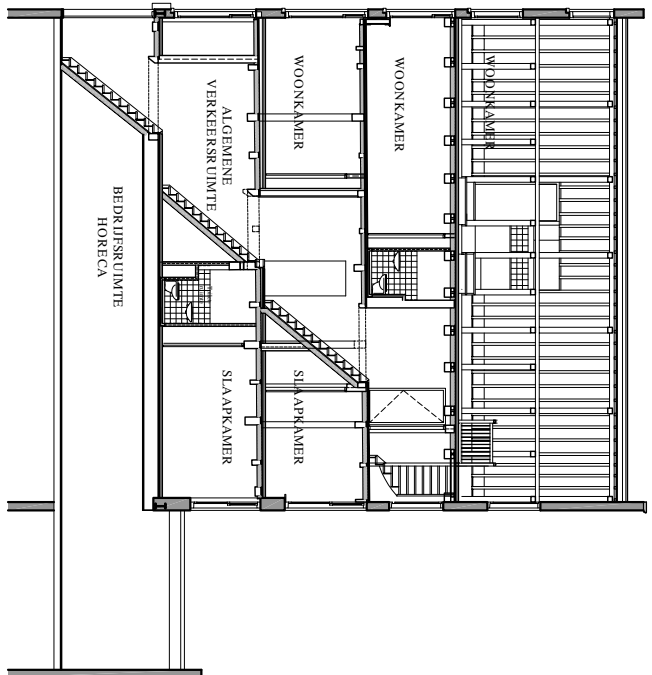
DOORSNEDEN A-A
