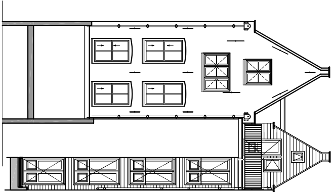
ACHTERGEVELS
