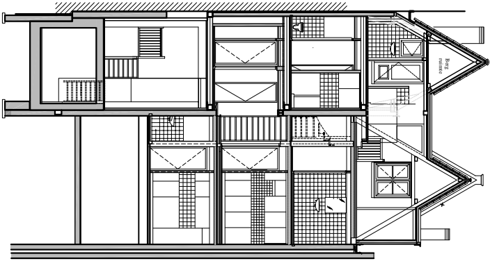
DOORSNEDEN C-C
