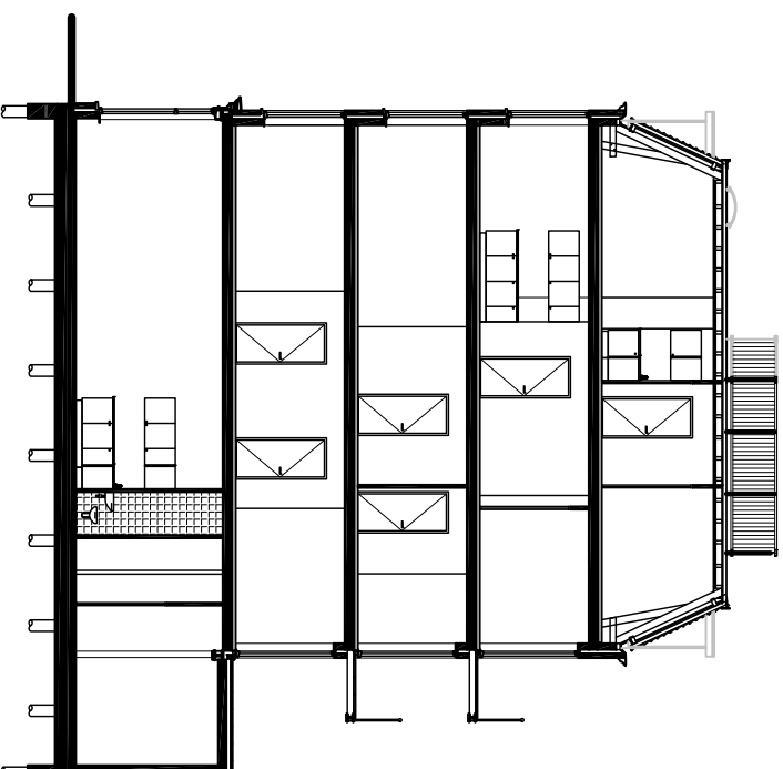
Doorsnede
