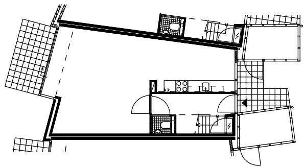
begane grond
