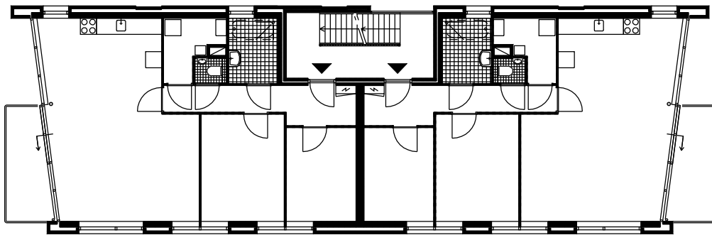
1e verdieping
