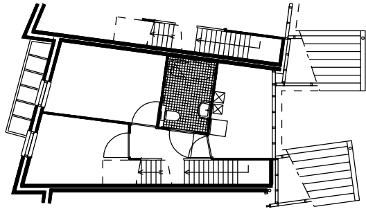
1e verdieping
