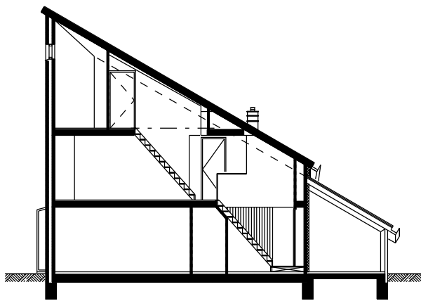
langsdoorsnede
