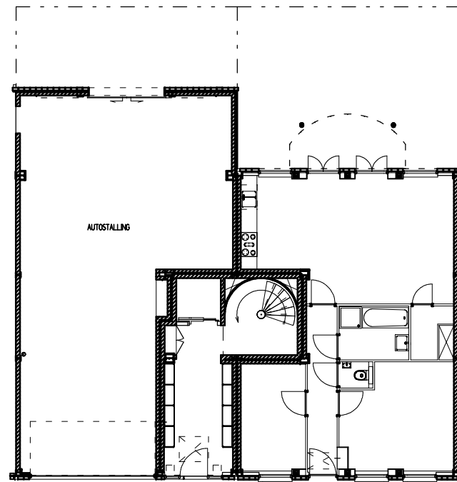
BEGANE GROND
