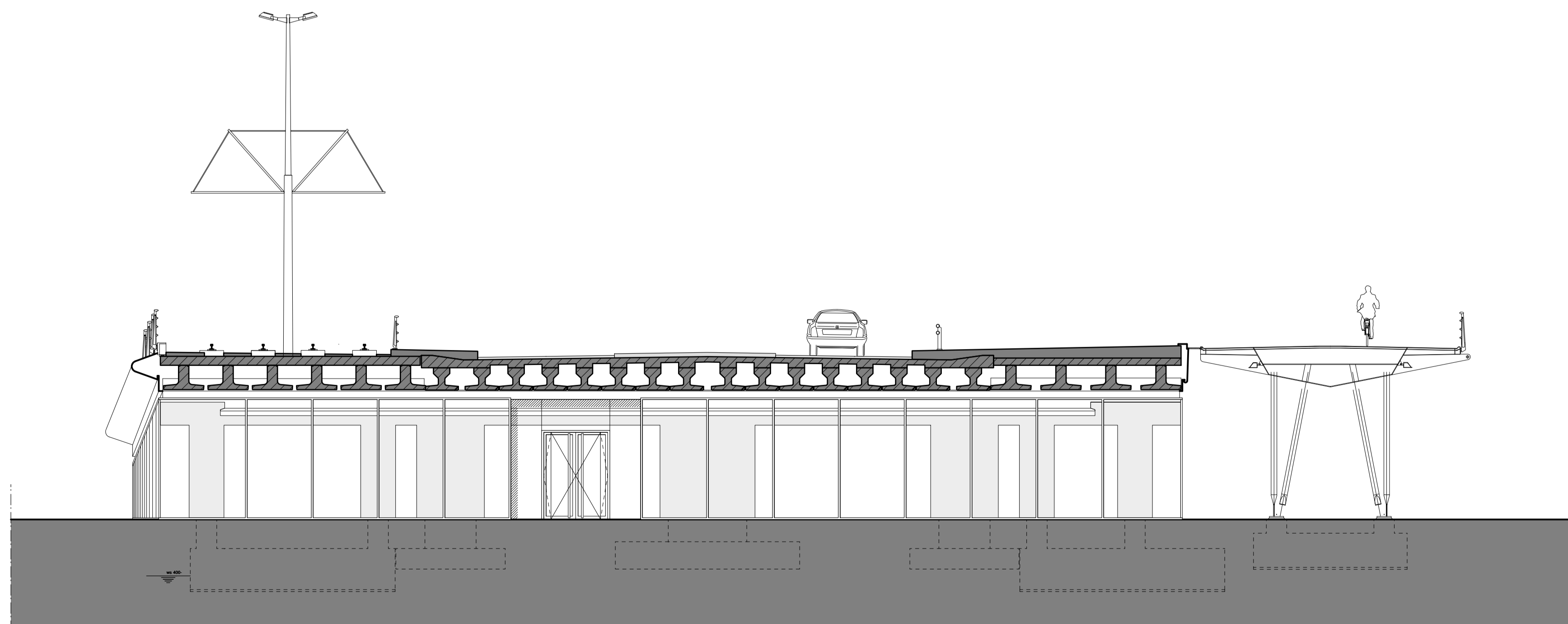
OOSTGEVEL; DOORSNEDE T.P.V. STRAMIEN 11
