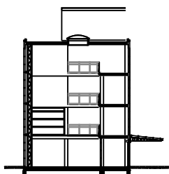
DOORSNEDE WINTERTUIN
