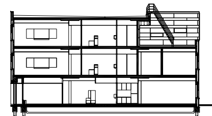
dwarsdoorsnede
