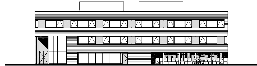
gevel Anderlechtlaan
