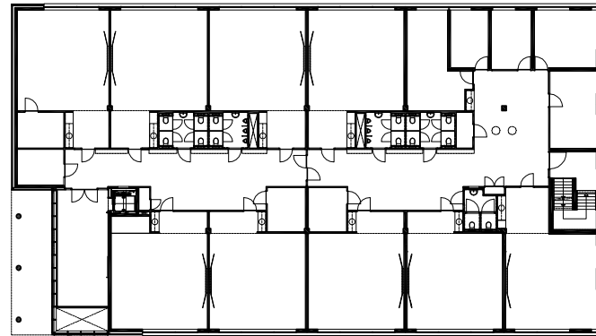
eerste verdieping
