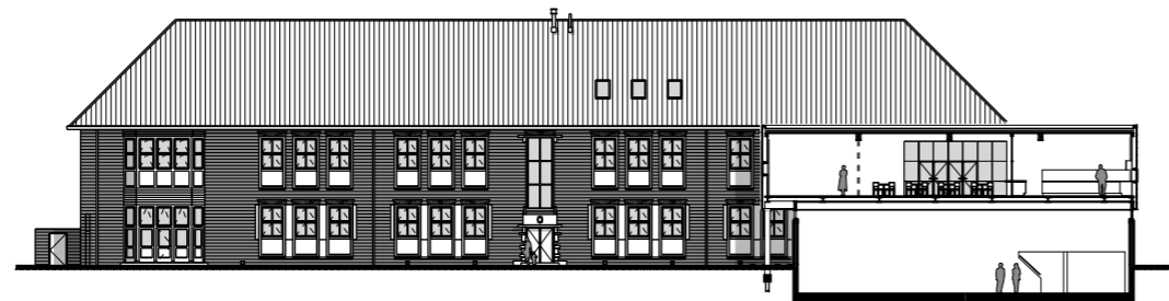
langsdoorsnede
