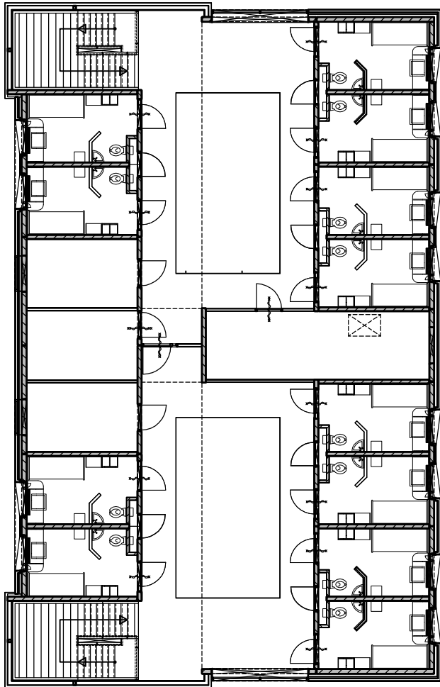
Plattegrond 2e verdieping
