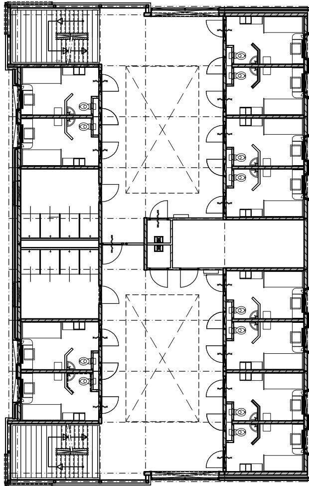
Plattegrond 1e verdieping
