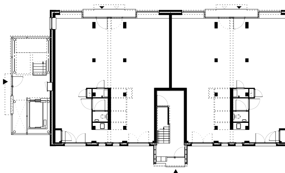
begane grond / bedrijfsruimten - blok 34
