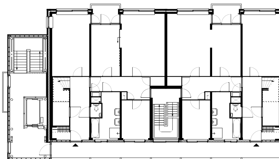
3e verdieping / entree maisonnettes - blok 30 / 34
