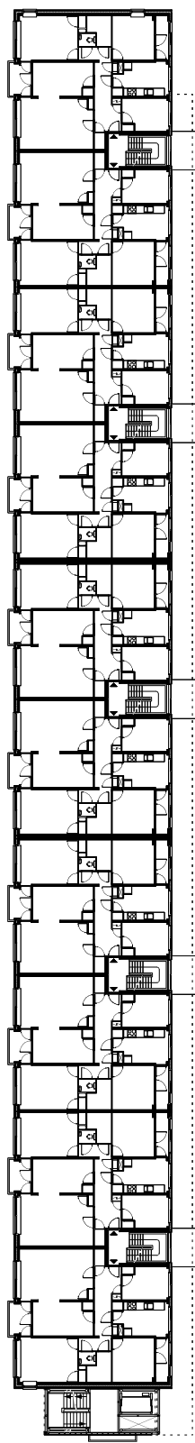
1e+2e verdieping - blok 30 / 34
