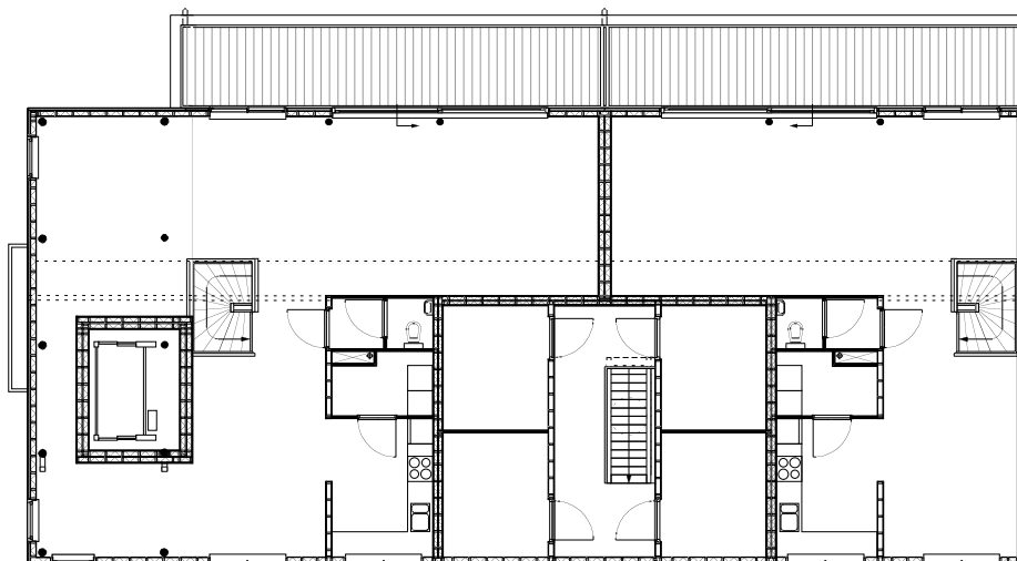
4e verdieping / verdieping maisonnettes - blok 30 / 34
