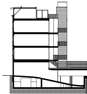
dwarsdoorsnede C
