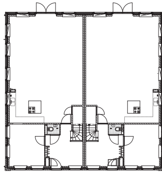
begane grond
