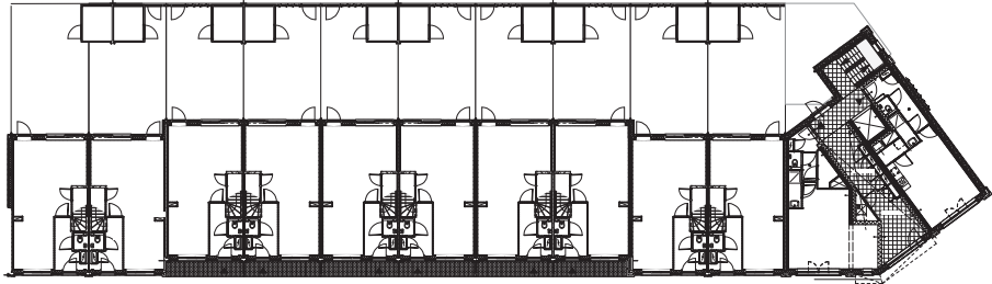
begane grond
