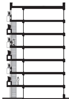
doorsnede
