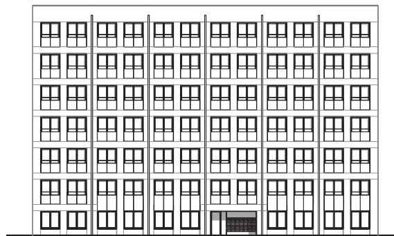
voorgevel
