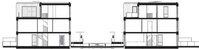
doorsnede
