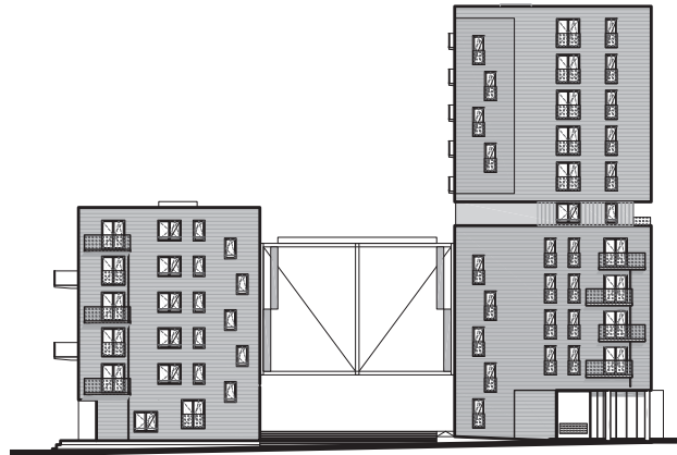
zuidgevel
