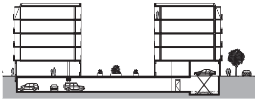
doorsnede
