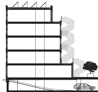
doorsnede
