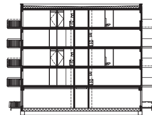
doorsnede
