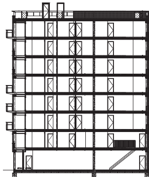
doorsnede
