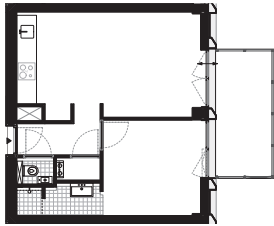
woning plattegrond (Sjuul)
