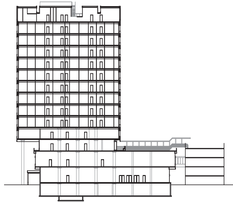
doorsnede
