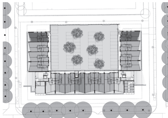
situatie met begane grond
