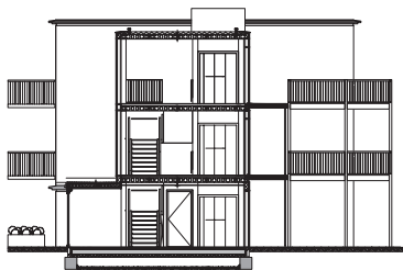
doorsnede
