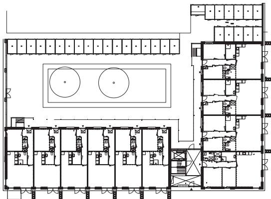
begane grond
