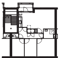
woning plattegrond
