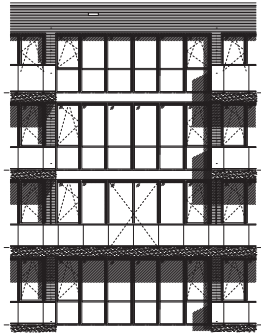
detail achtergevel
