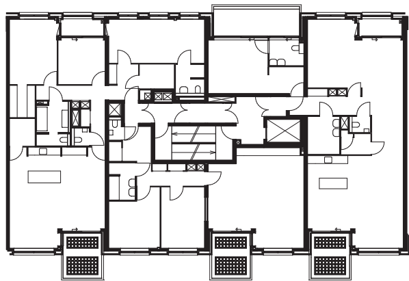
zesde verdieping
