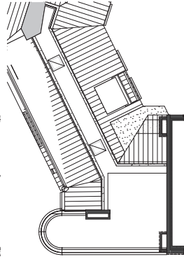
derde verdieping
