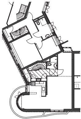
eerste verdieping
