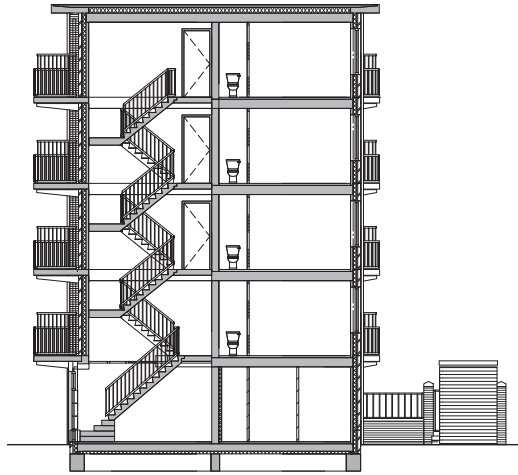
doorsnede AA
