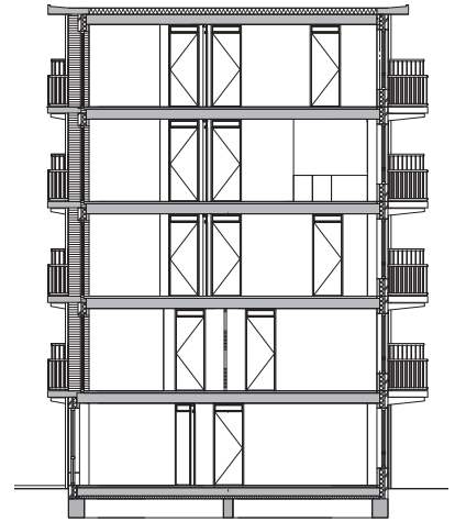
doorsnede BB
