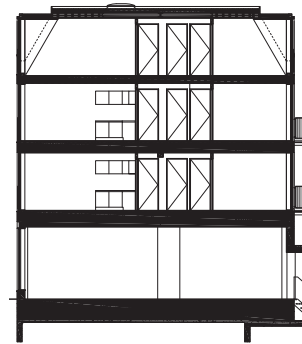
doorsnede
