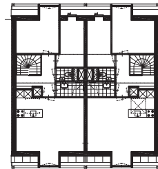
kapverdieping
