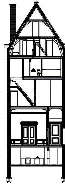
doorsnede
