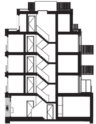
doorsnede
