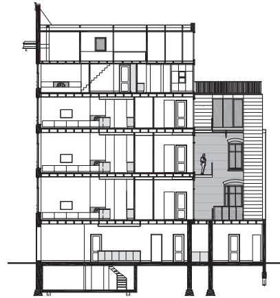
doorsnede
