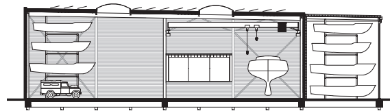
dwarsdoorsnede
