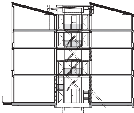
doorsnede
