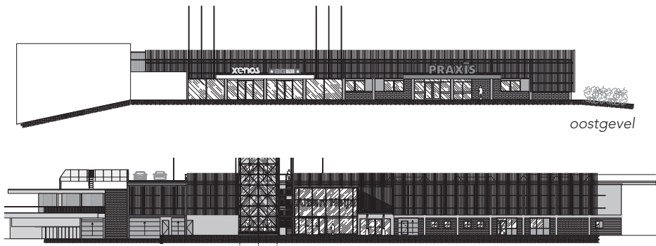
zuidgevel
