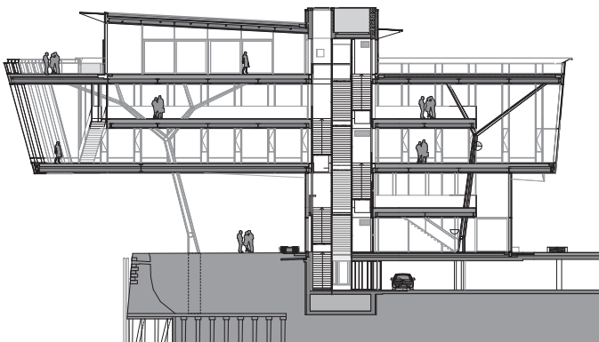
langsdoorsnede
