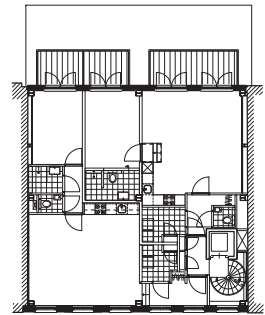
tweede verdieping
