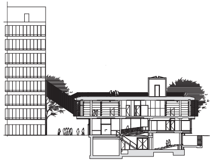
dwarsdoorsnede
