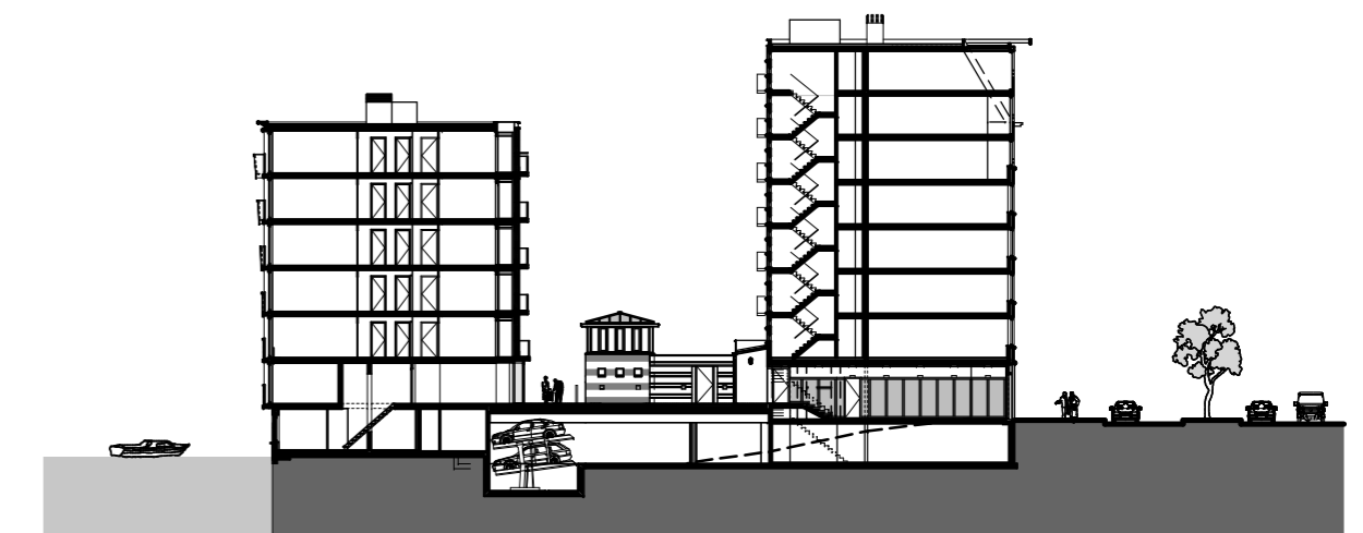
Doorsnede 1:500
