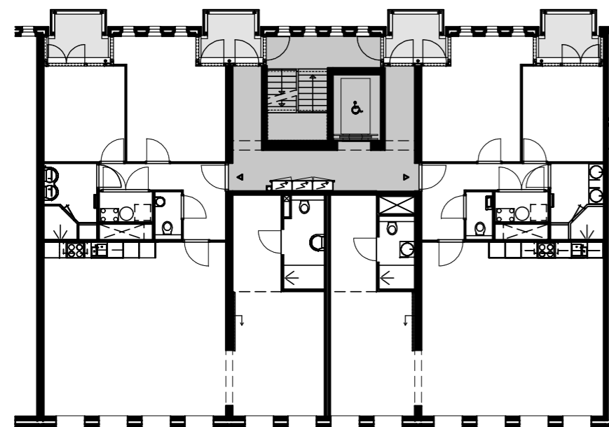
Valkenburgerstraat 1:200
