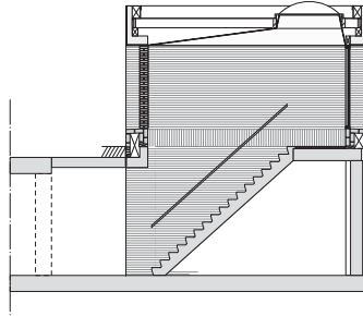
doorsnede
