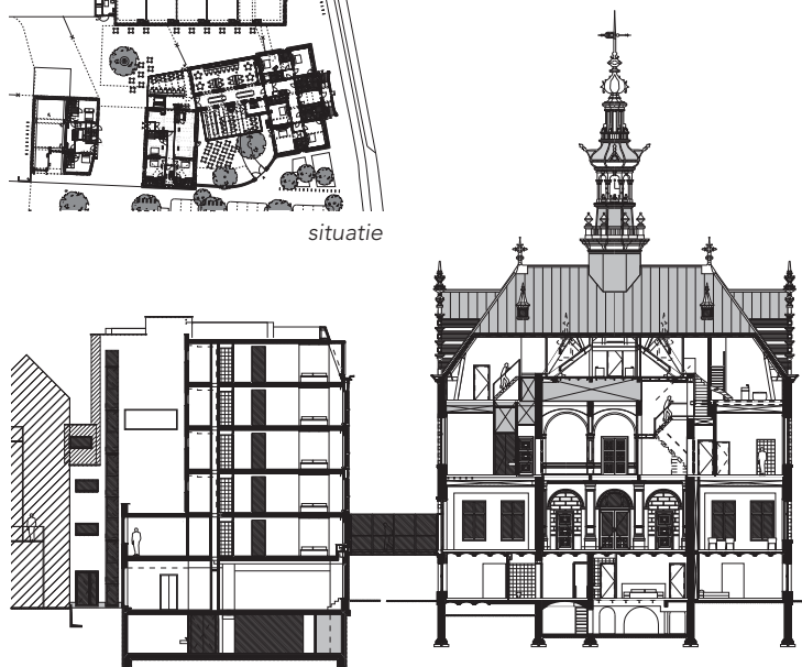
doorsnede
