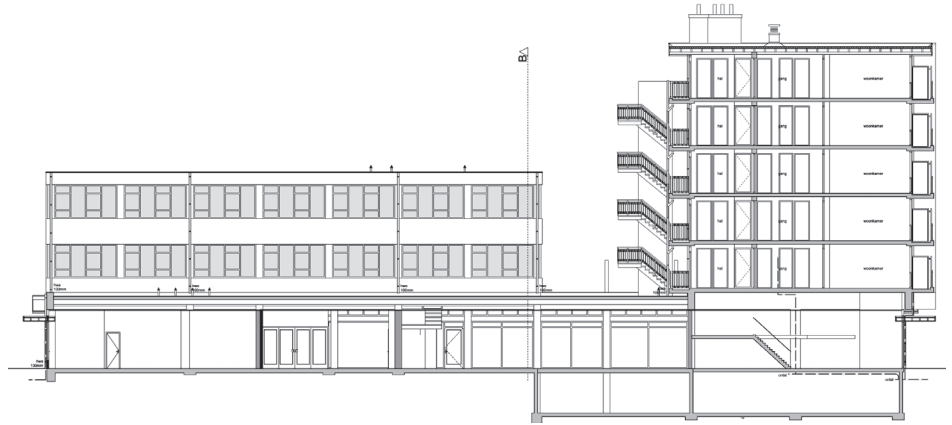
doorsnede
