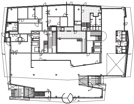
begane grond
