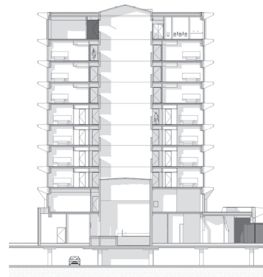
doorsnede
